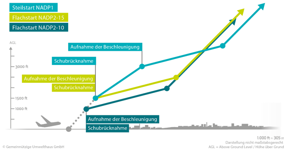
Infografik Erläuterung Steilstart- und Flachstartverfahren
