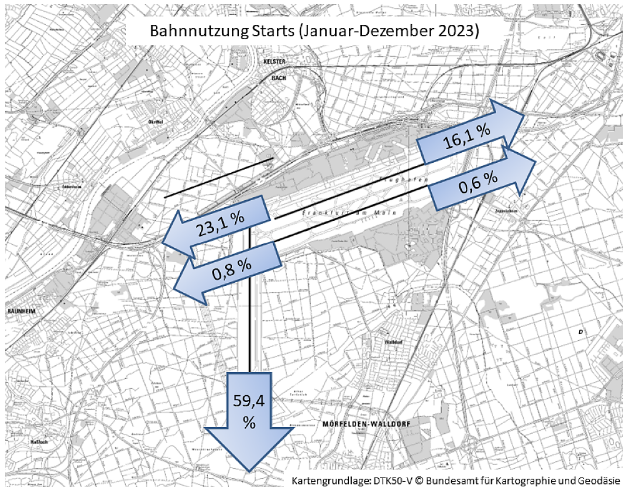
Bahnverteilung Starts (FRA) (Januar-Dezember 2023)
